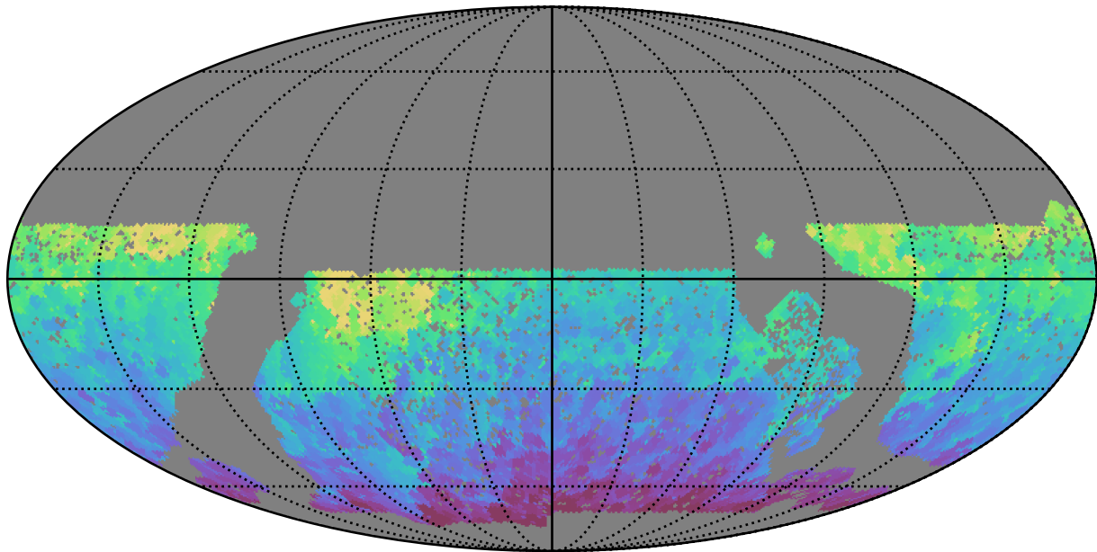
baseline_v3.0_10yrs WFD z band: Min HA
