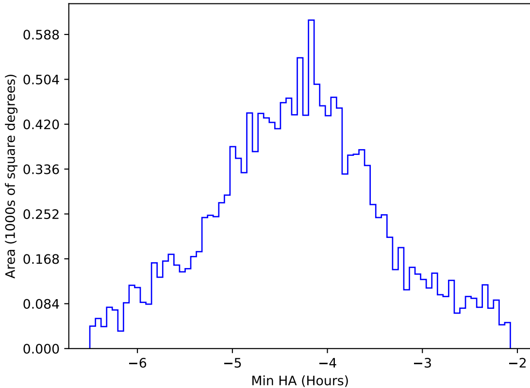
baseline_v3.0_10yrs WFD z band: Min HA
