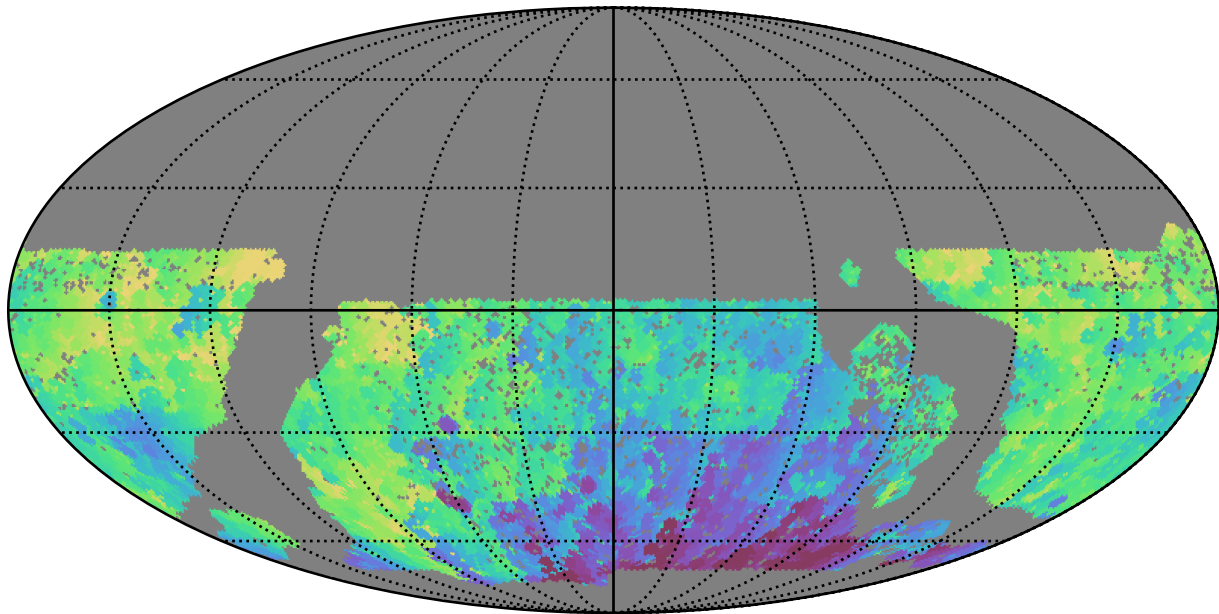
baseline_v3.0_10yrs WFD y band: Min HA
