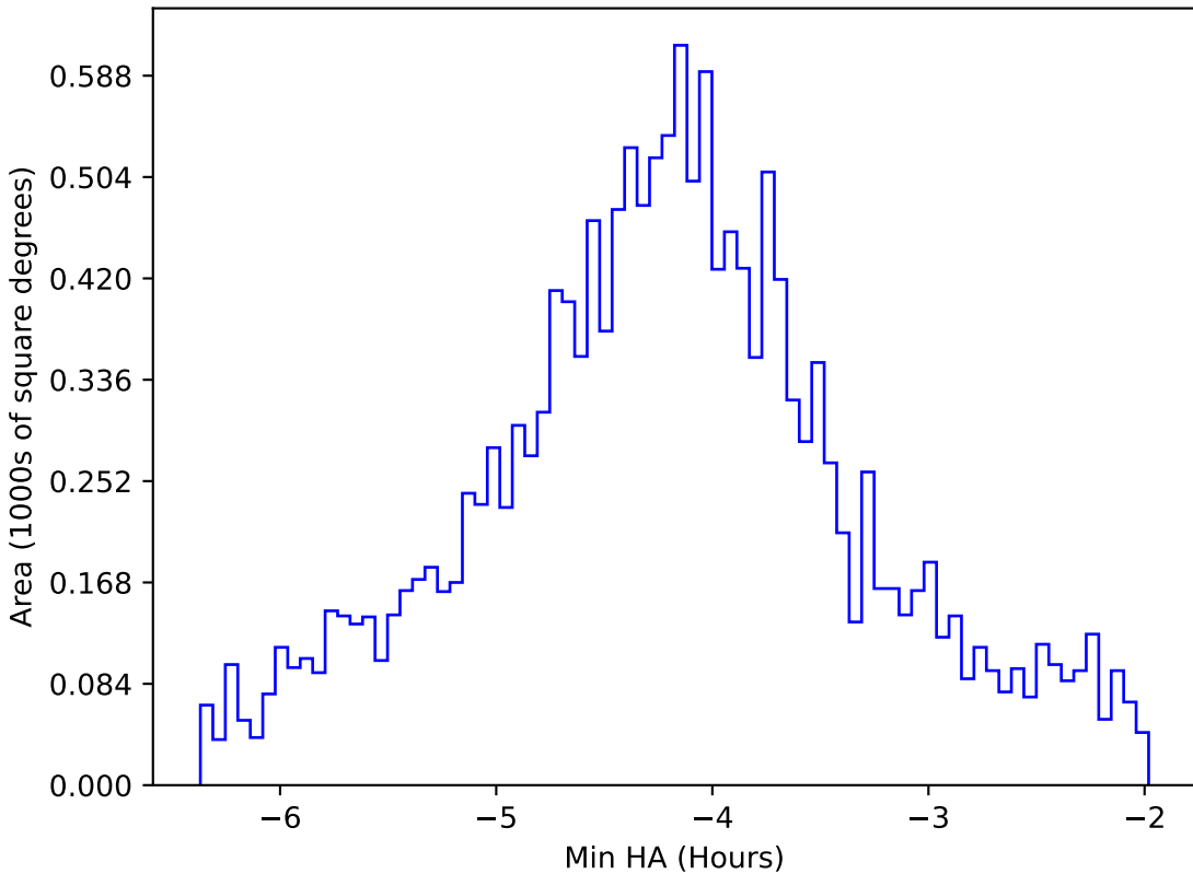
baseline_v3.0_10yrs WFD i band: Min HA
