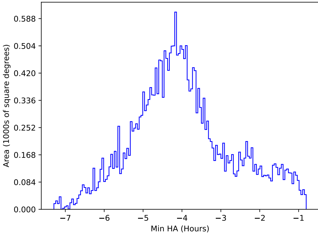
baseline_v3.0_10yrs All sky z band: Min HA
