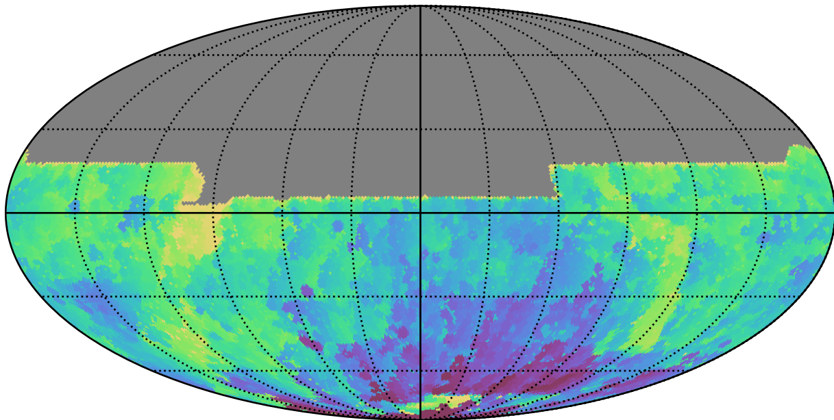
baseline_v3.0_10yrs All sky y band: Min HA
