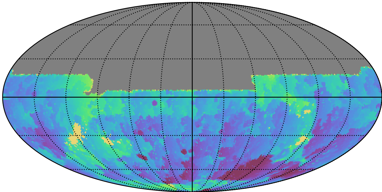
baseline_v3.0_10yrs All sky u band: Min HA
