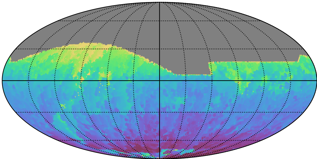
baseline_v3.0_10yrs All sky r band: Min HA
