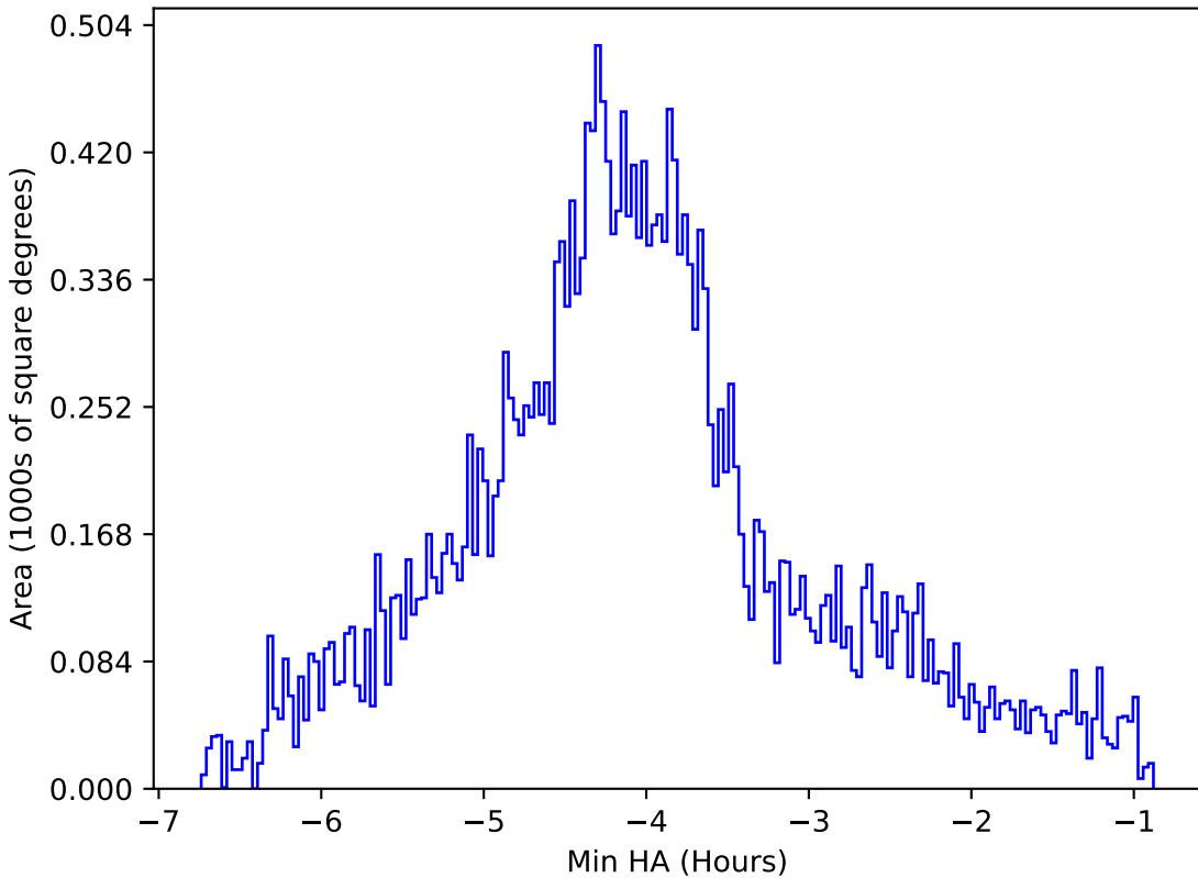
baseline_v3.0_10yrs All sky r band: Min HA
