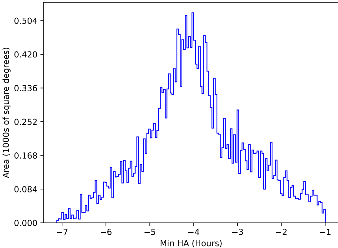
baseline_v3.0_10yrs All sky i band: Min HA
