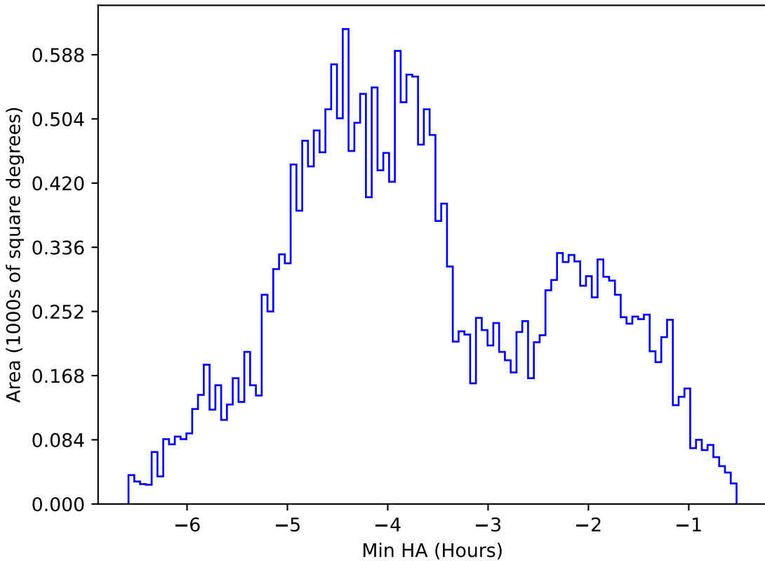
baseline_v3.0_10yrs All sky g band: Min HA
