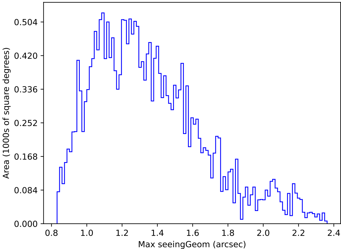
baseline_v3.0_10yrs Yr 1 y band: Max seeingGeom
