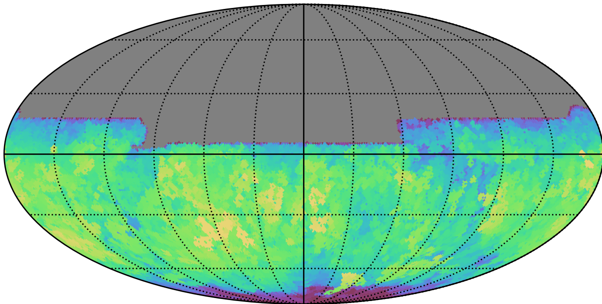
baseline_v3.0_10yrs All sky y band: Max saturation_mag
