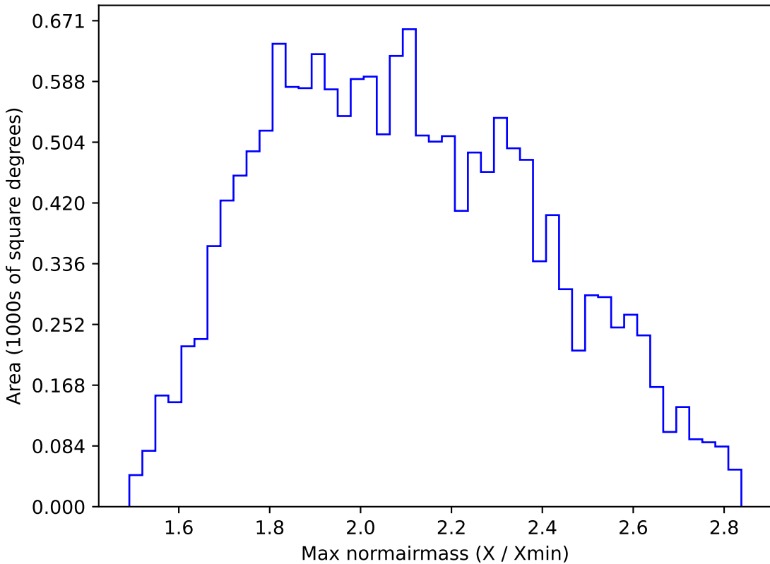
baseline_v3.0_10yrs WFD y band: Max normairmass
