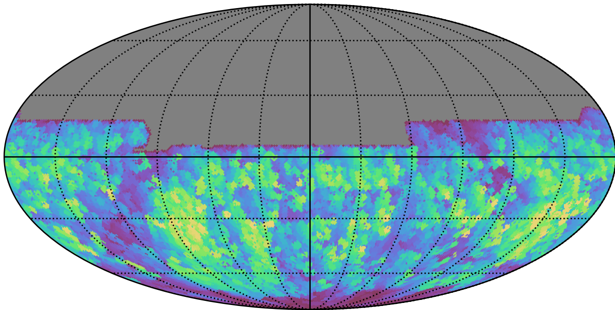
baseline_v3.0_10yrs All sky y band: Max normairmass
