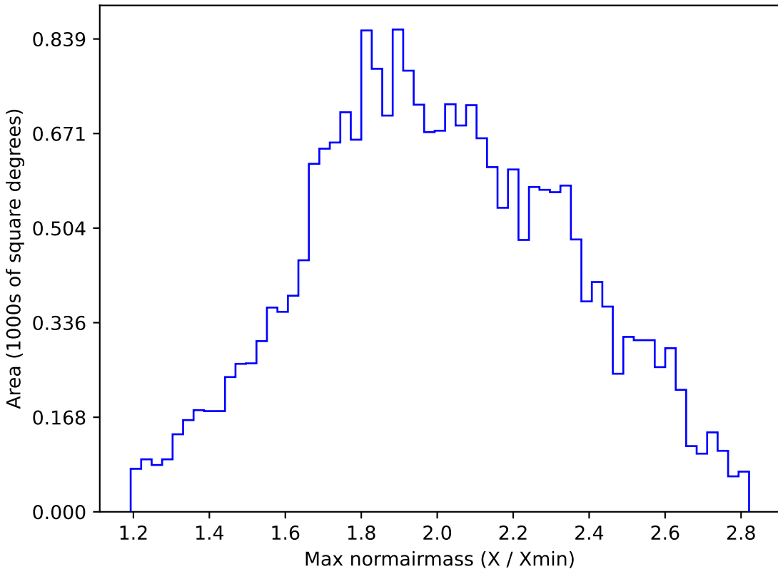
baseline_v3.0_10yrs All sky y band: Max normairmass
