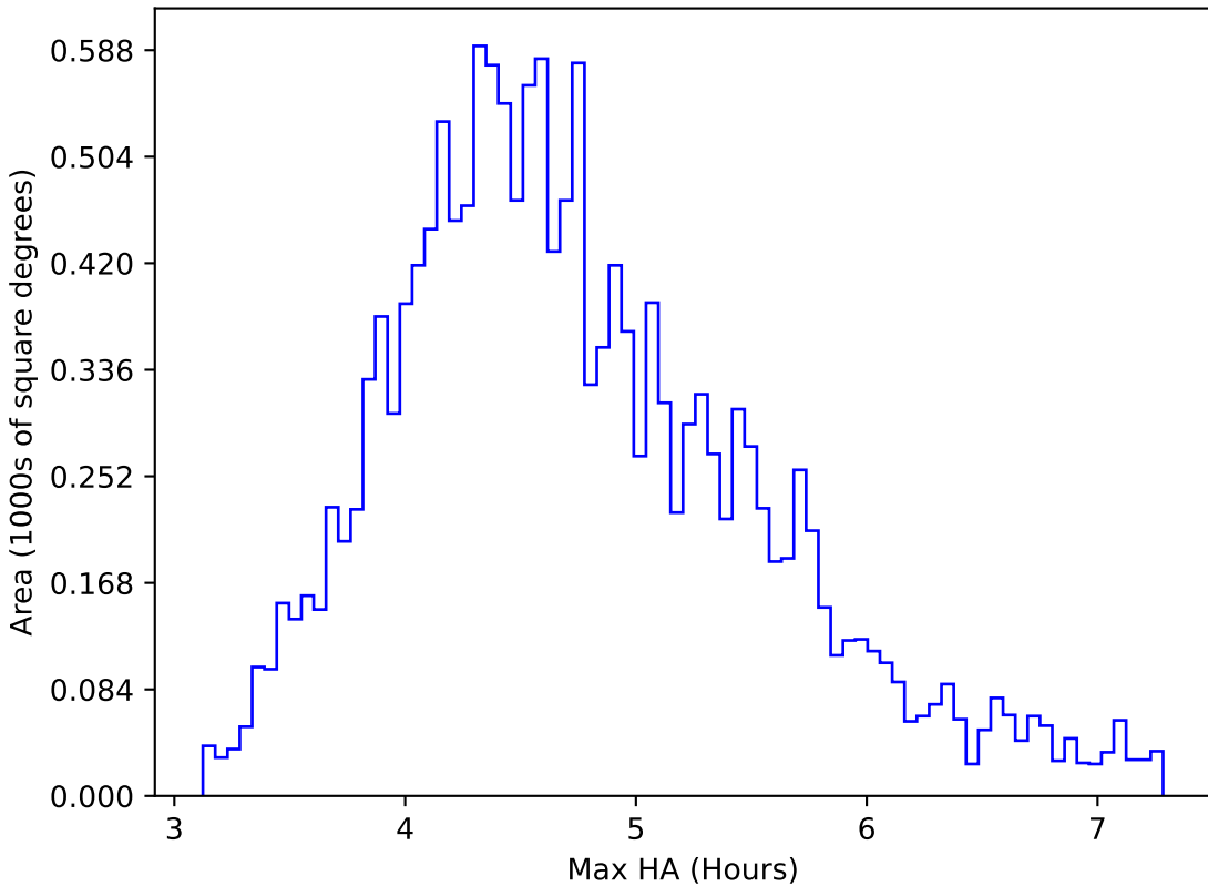
baseline_v3.0_10yrs WFD y band: Max HA
