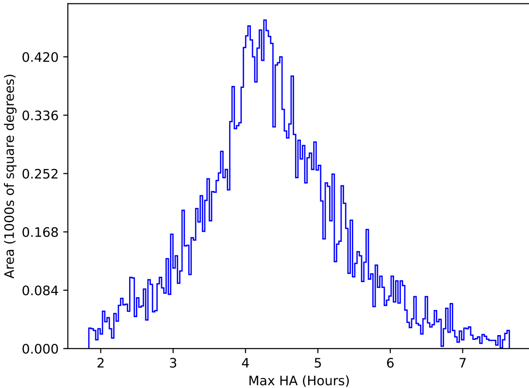
baseline_v3.0_10yrs All sky z band: Max HA
