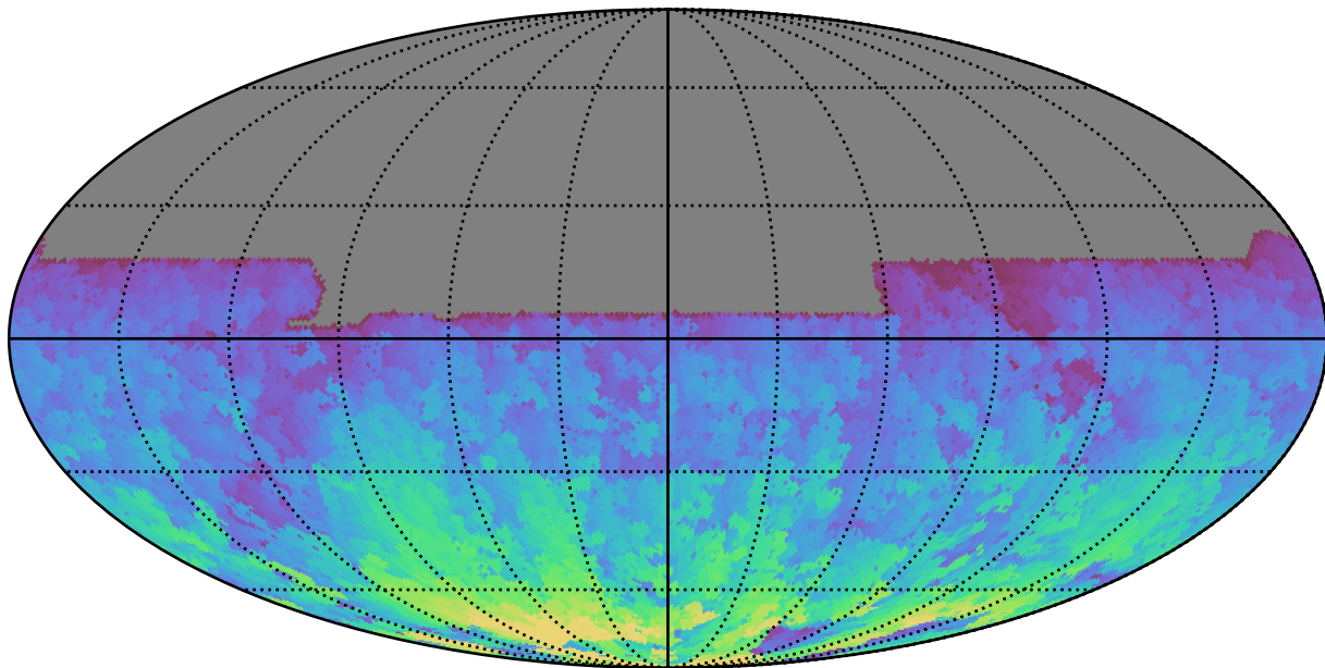
baseline_v3.0_10yrs All sky y band: Max HA
