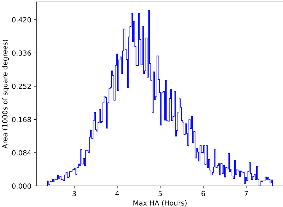
baseline_v3.0_10yrs All sky y band: Max HA
