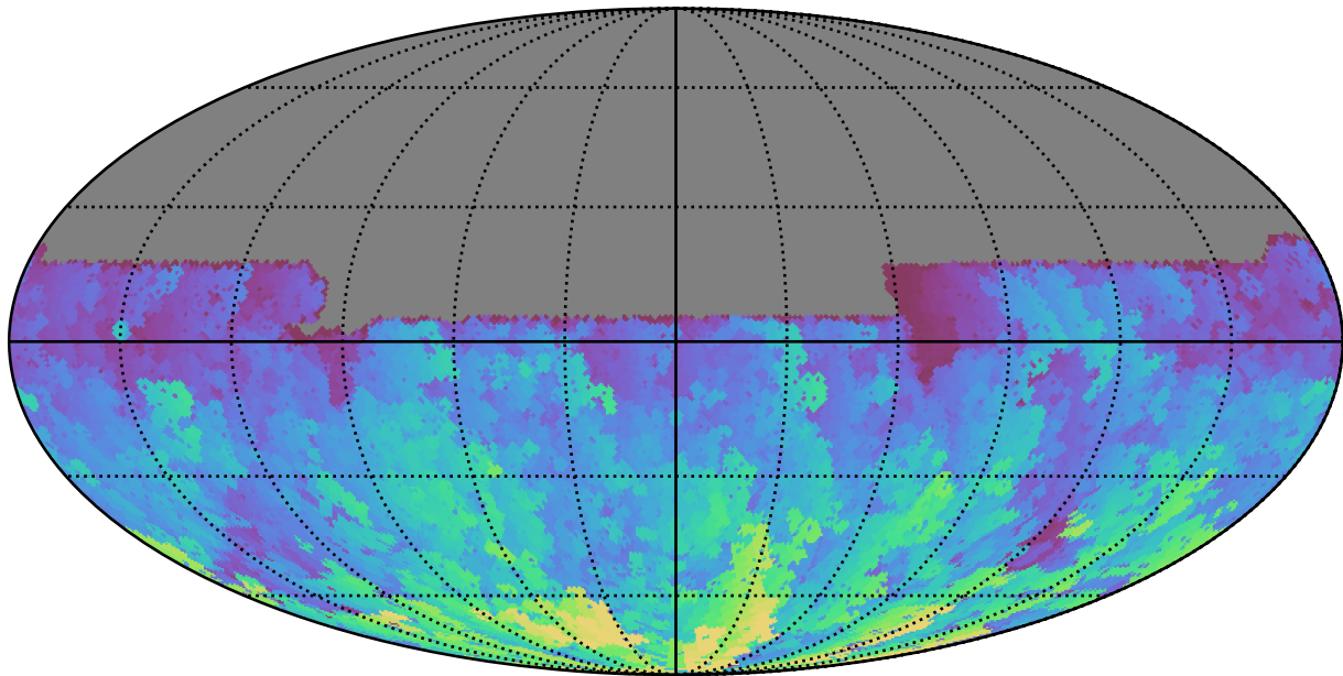
baseline_v3.0_10yrs All sky u band: Max HA
