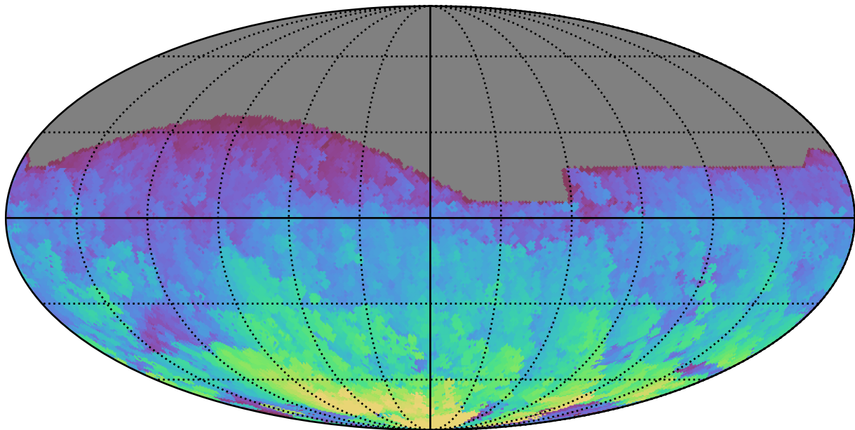
baseline_v3.0_10yrs All sky r band: Max HA
