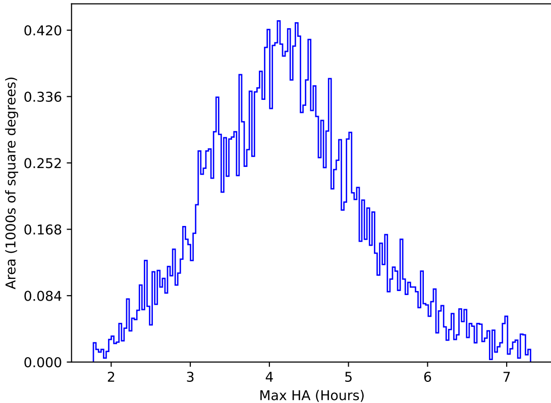
baseline_v3.0_10yrs All sky r band: Max HA
