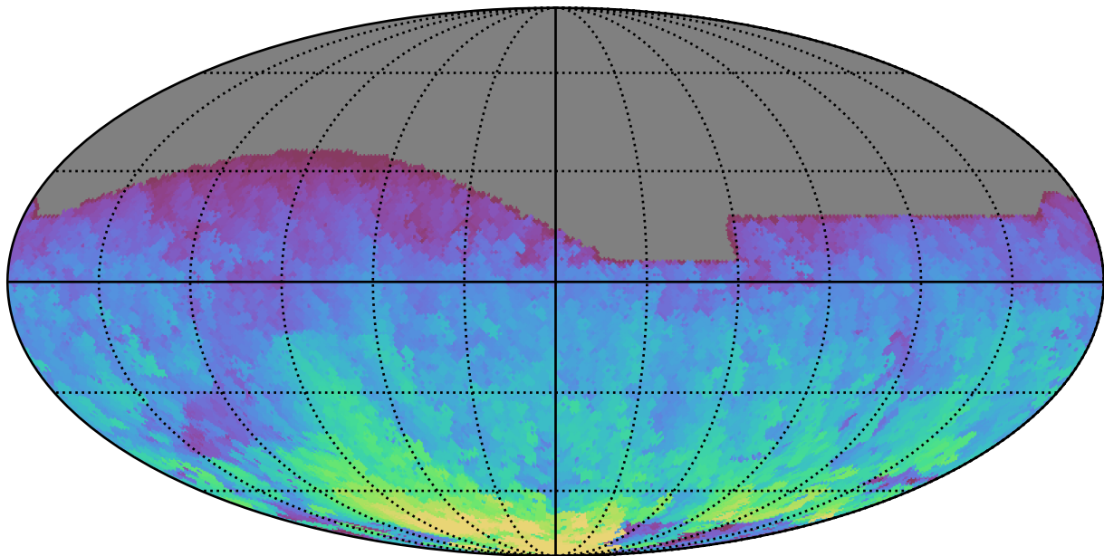
baseline_v3.0_10yrs All sky i band: Max HA
