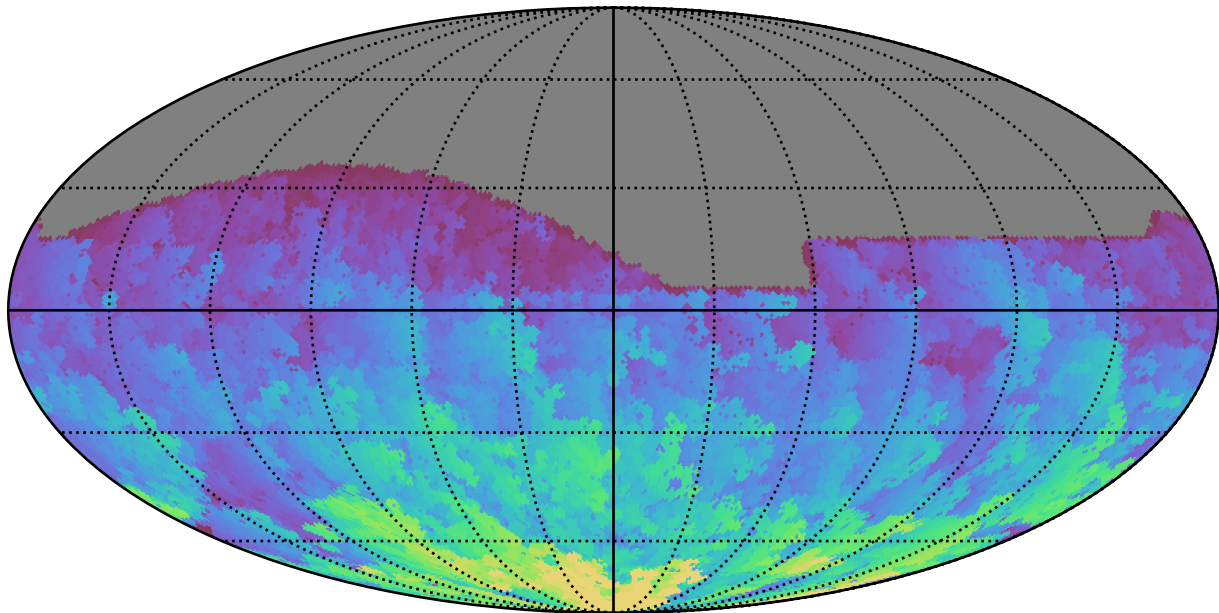
baseline_v3.0_10yrs All sky g band: Max HA
