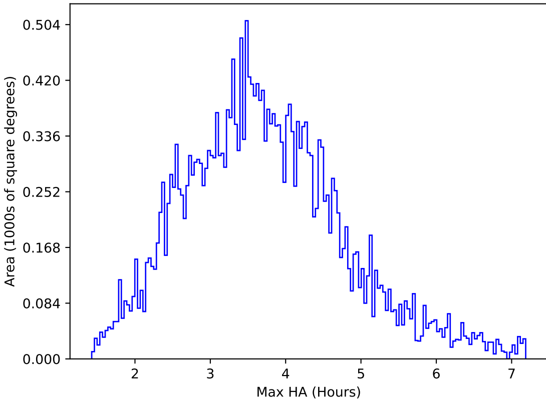
baseline_v3.0_10yrs All sky g band: Max HA
