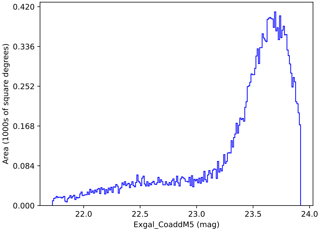
baseline_v3.0_10yrs Yr 1 y band: Exgal_CoaddM5
