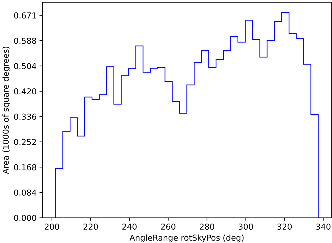
baseline_v3.0_10yrs WFD y band: AngleRange rotSkyPos
