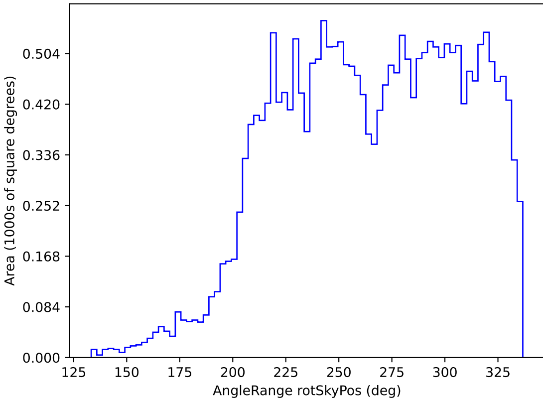
baseline_v3.0_10yrs All sky y band: AngleRange rotSkyPos
