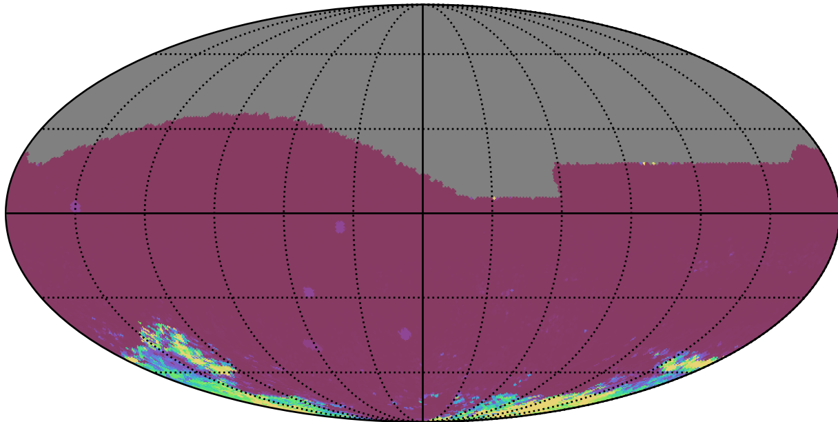
baseline_v3.0_10yrs All sky iz bands: 75th Percentile Intranight Timespan
