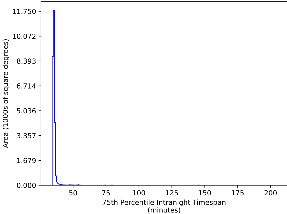
baseline_v3.0_10yrs All sky iz bands: 75th Percentile Intranight Timespan
