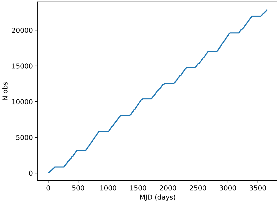
baseline_v3.0_10yrs note like DD:ELAISS1%: Cumulative
