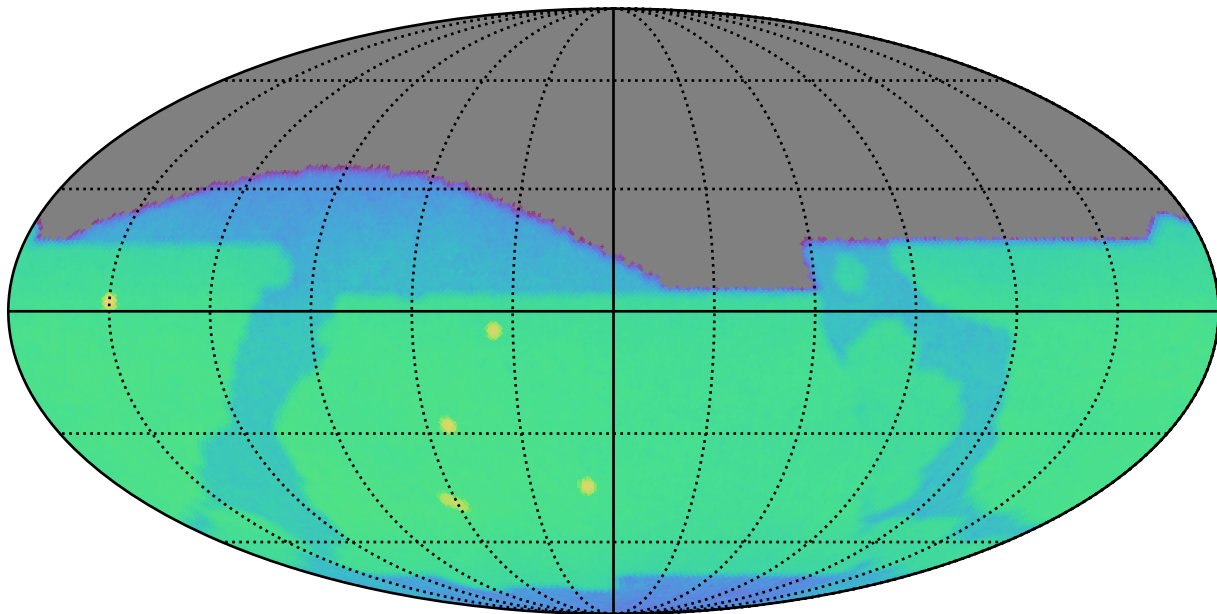
baseline_v3.0_10yrs z: CoaddM5
