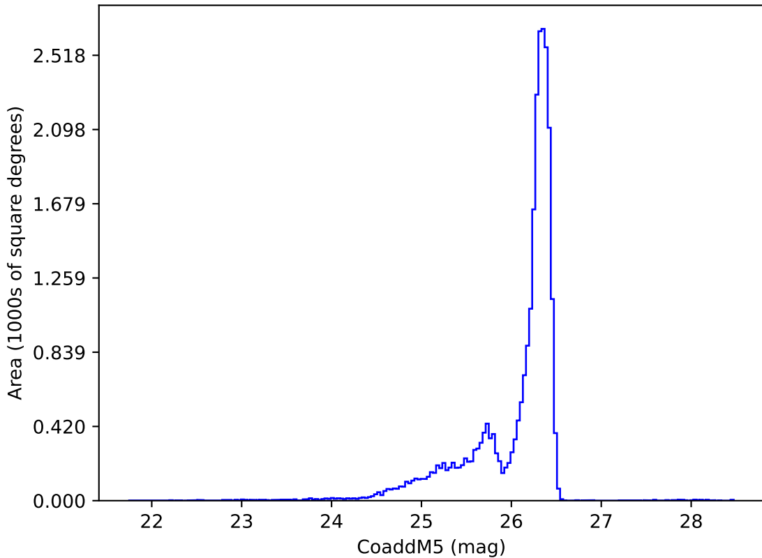
baseline_v3.0_10yrs i: CoaddM5
