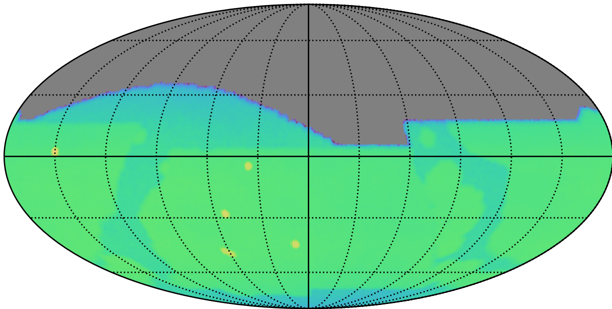
baseline_v3.0_10yrs : CoaddM5
