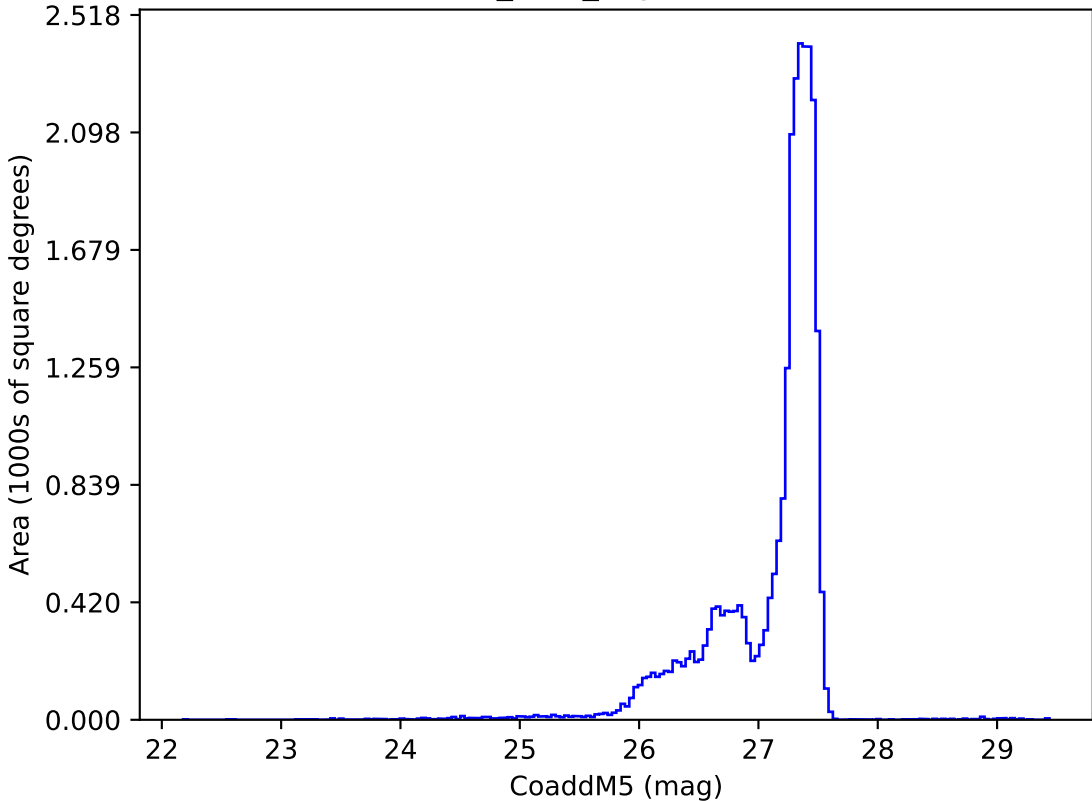
baseline_v3.0_10yrs : CoaddM5
