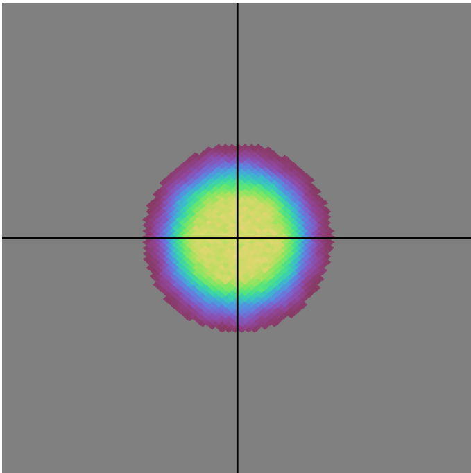
baseline_v3.0_10yrs r band: DD:XMM_LSS NVisits
