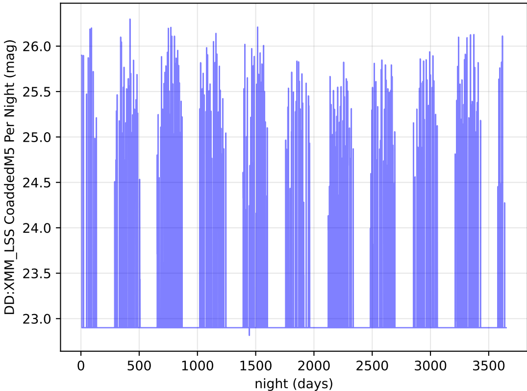
baseline_v3.0_10yrs r band: DD:XMM_LSS CoaddedM5 Per Night
