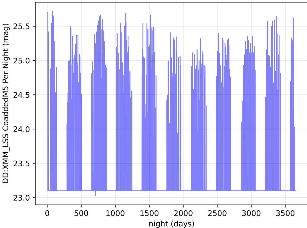
baseline_v3.0_10yrs i band: DD:XMM_LSS CoaddedM5 Per Night
