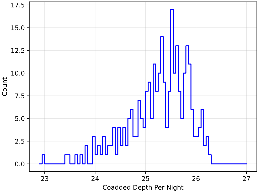
baseline_v3.0_10yrs r band: DD:XMM_LSS CoaddM5PerNight
