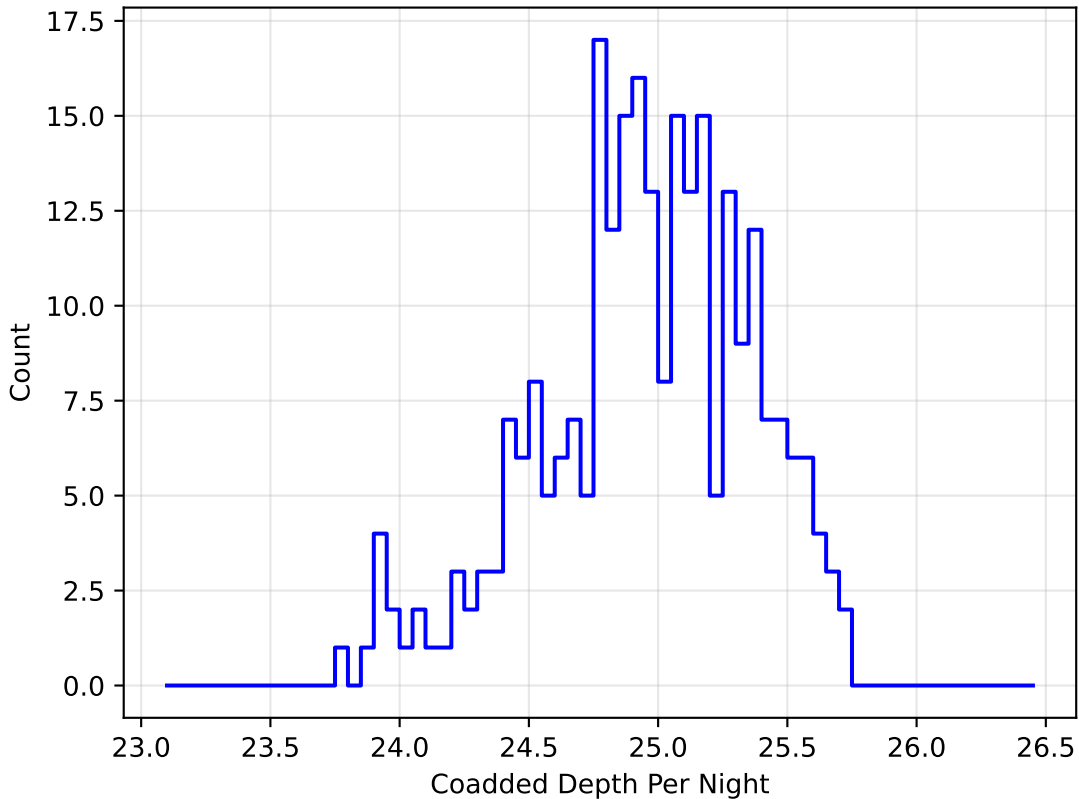
baseline_v3.0_10yrs i band: DD:XMM_LSS CoaddM5PerNight
