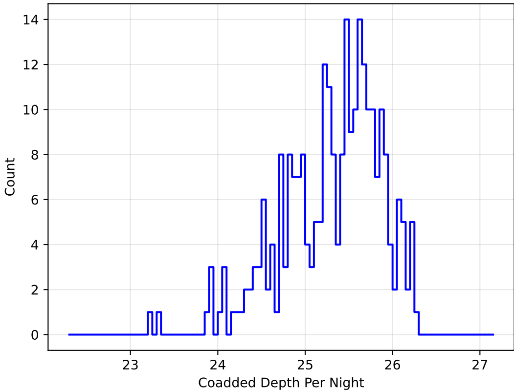
baseline_v3.0_10yrs g band: DD:XMM_LSS CoaddM5PerNight
