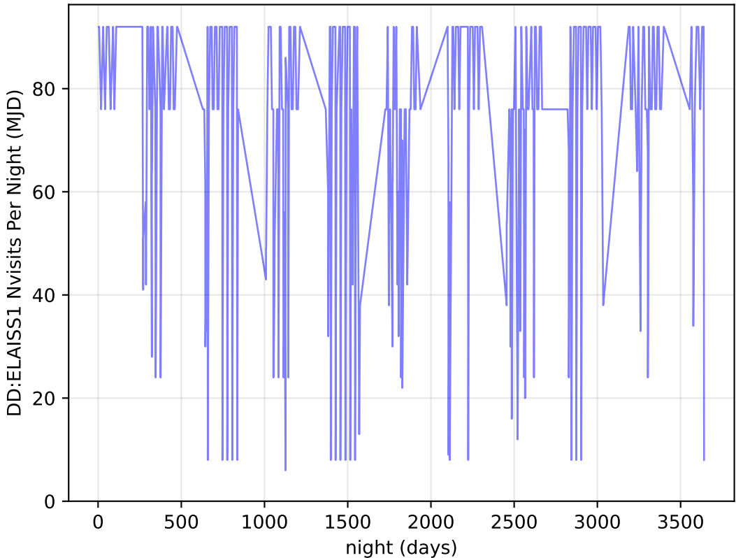
baseline_v3.0_10yrs all bands: DD:ELAISS1 Nvisits Per Night
