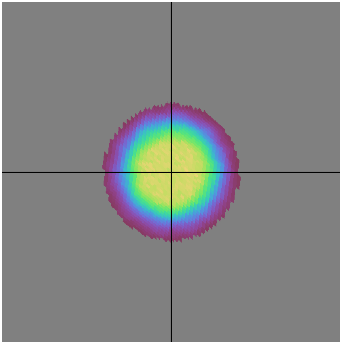
baseline_v3.0_10yrs r band: DD:ELAISS1 NVisits
