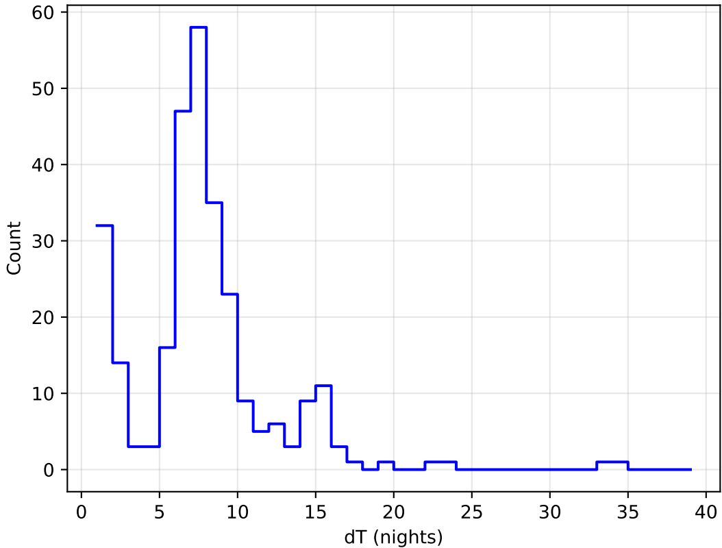
baseline_v3.0_10yrs all bands: DD:ELAISS1 Delta Nights Histogram
