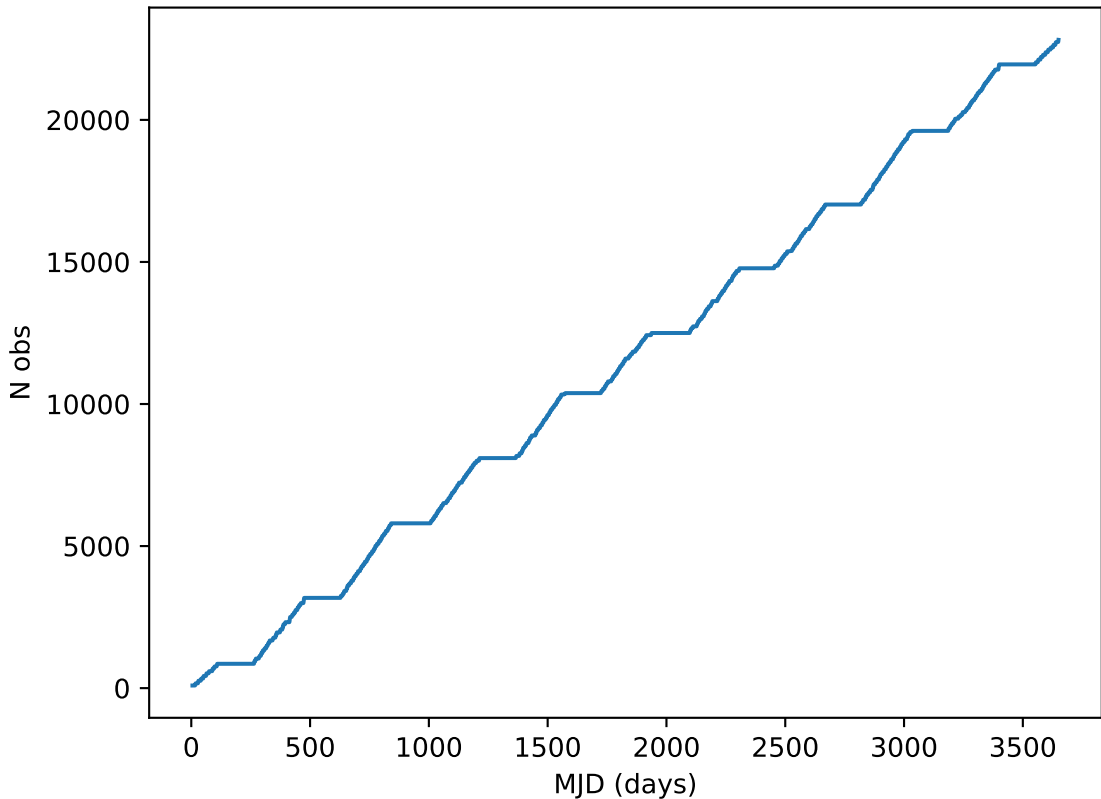
baseline_v3.0_10yrs all bands: DD:ELAISS1 Cumulative NVisits
