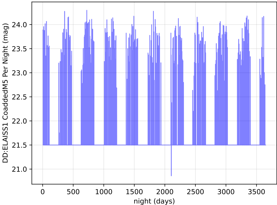
baseline_v3.0_10yrs y band: DD:ELAISS1 CoaddedM5 Per Night
