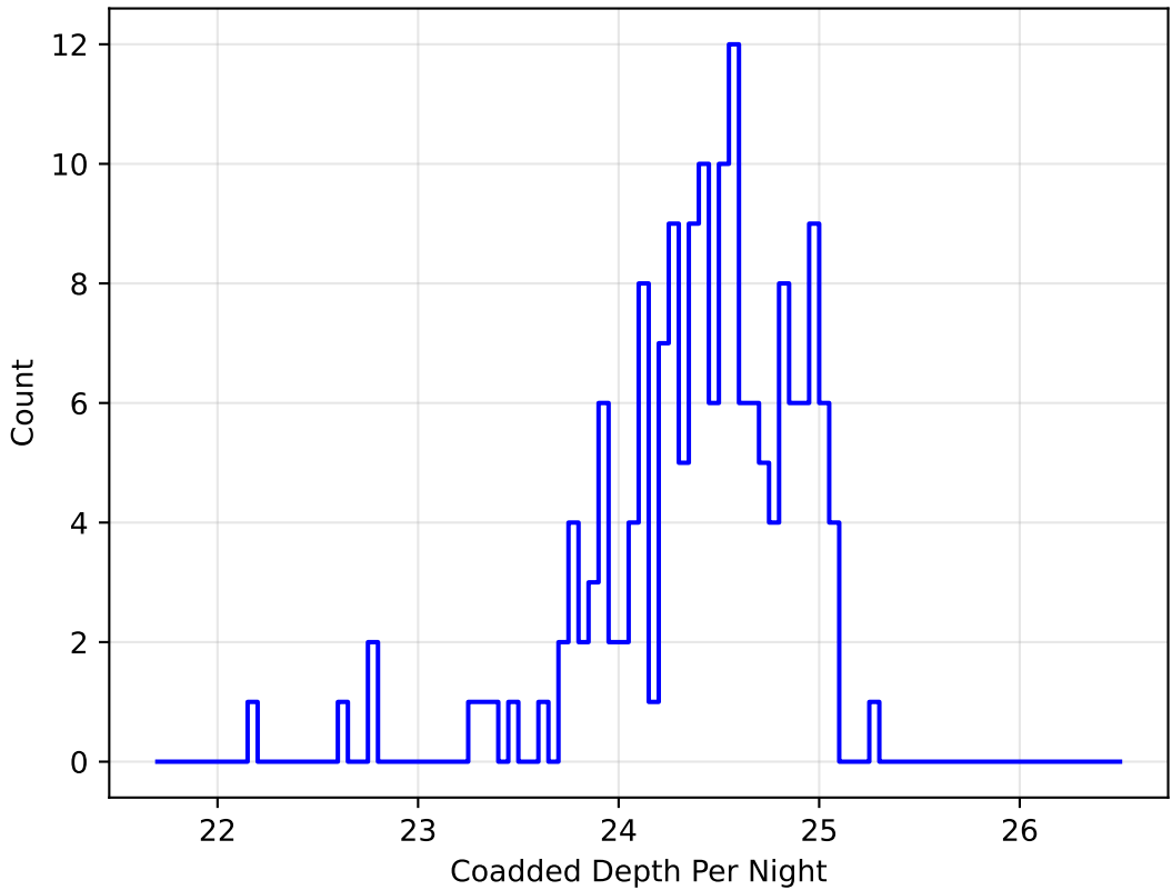
baseline_v3.0_10yrs z band: DD:ELAISS1 CoaddM5PerNight
