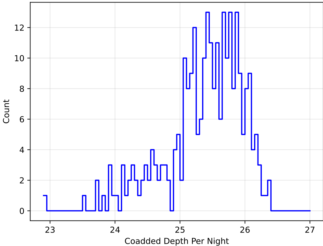
baseline_v3.0_10yrs r band: DD:ELAISS1 CoaddM5PerNight
