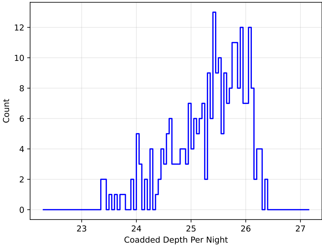
baseline_v3.0_10yrs g band: DD:ELAISS1 CoaddM5PerNight
